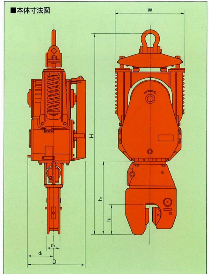
■ 本体寸法表 (単位: mm)
